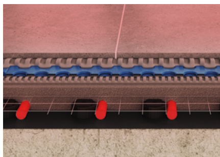
Укладка Mapeguard UM 35 на теплый пол
