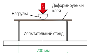
1. Испытательный стенд для измерения эластичности тонкого слоя клея в соответствии с его деформацией
